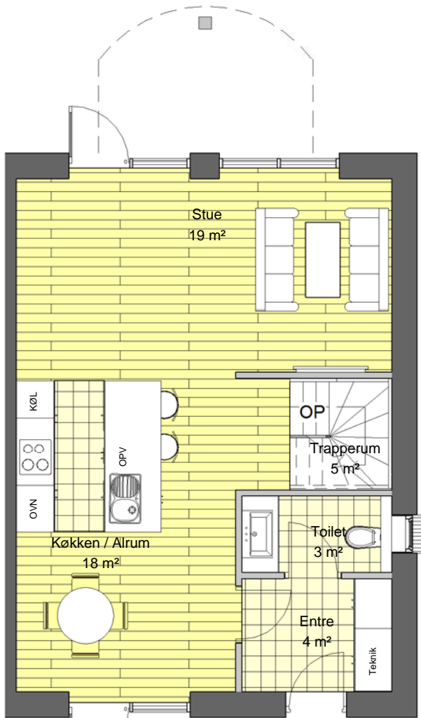
Stueplan
